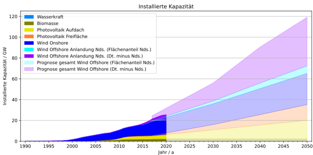
Abbildung 6: Installierte Kapazitäten von Wasserkraft, Biomasse, Photovoltaik, Wind Onshore und Wind Offshore. Bei Wind Offshore wurde bis 2020 die in Niedersachsen angelandete Kapazität dargestellt. Für die Prognose wurden im Vergleich dazu die bundesweiten Wind Offshore Kapazitäten aufgetragen
