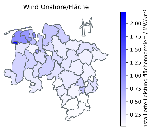
Abbildung 8: Installierte Wind Onshore Leistung flächennormiert bezogen auf Landkreise und kreisfreie Städte
