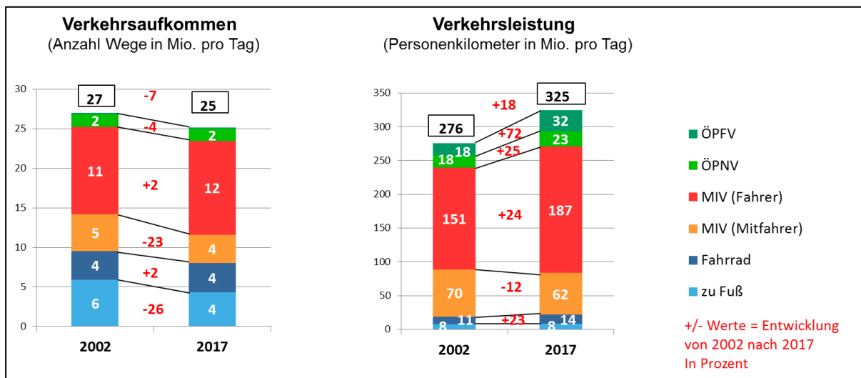
Abbildung 1: Entwicklung von Verkehrsaufkommen und Verkehrsleistung nach Verkehrsmitteln in Niedersachsen
