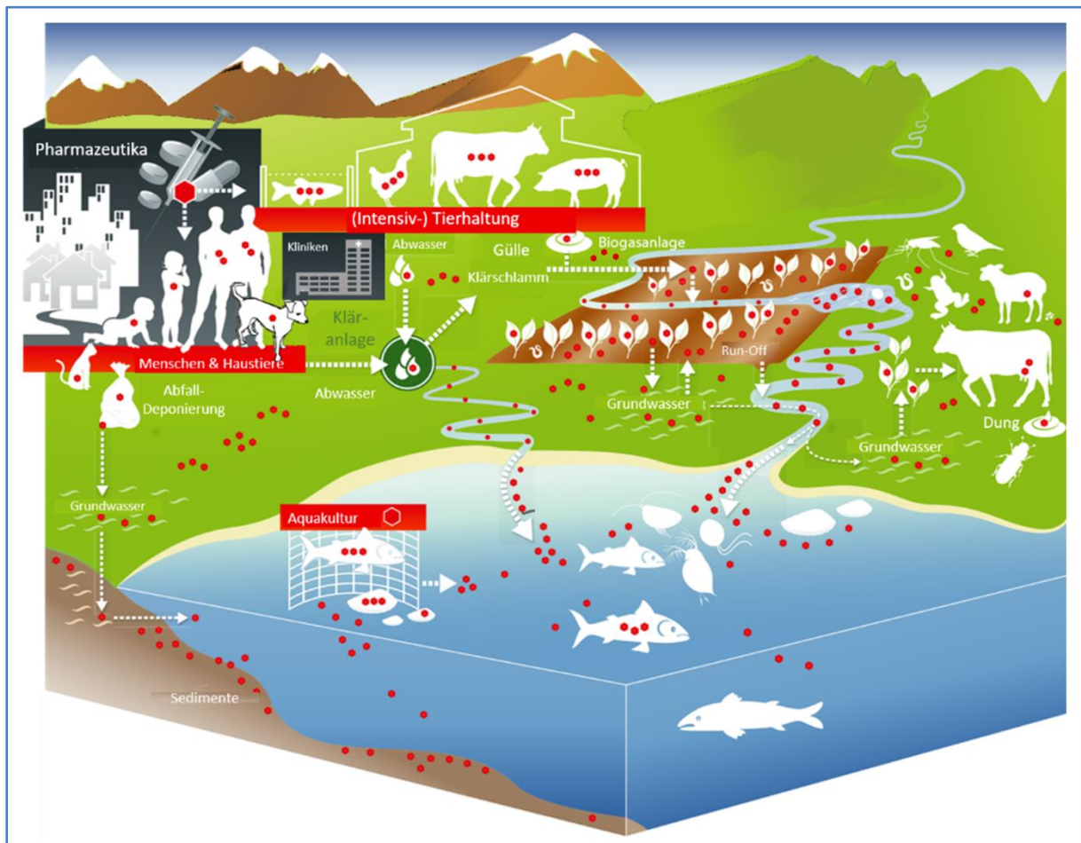
Abbildung 1. Eintragspfade von Antibiotika (schematisch als rote Punkte dargestellt) aus Human- und Tiermedizin in die Umwelt [27,33].
